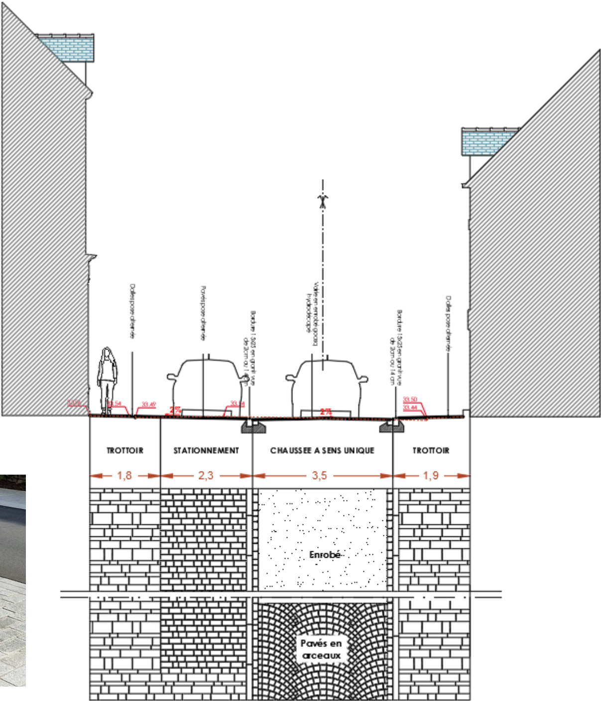
Stationnements longitudinaux : Pavés en granit
